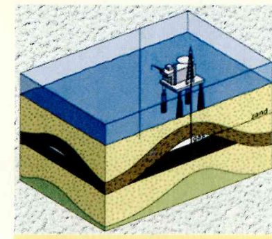
(fig B) Op deze dode zeediertjes stapelen lagen klei en zand zich op. Dit proces gaat vele miljoenen jaren door en uiteindelijk ontstaat aardolie.
