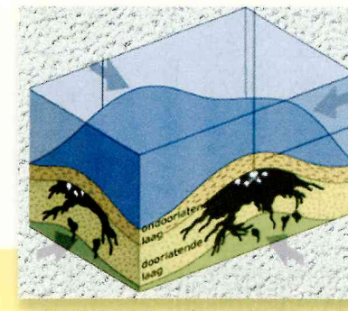
(fig C) Vanuit de ondergrond zoekt de olie een weg naar boven.
