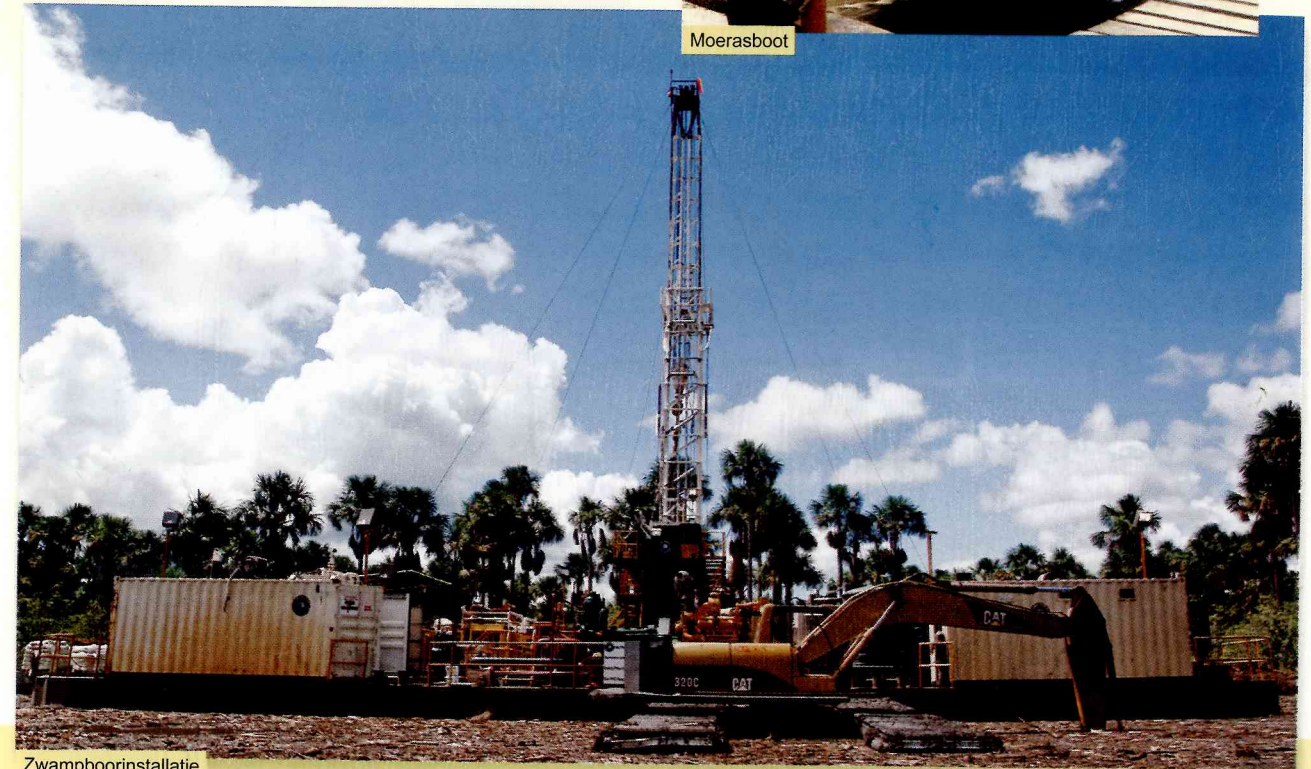
Zwampboorinstallatie
