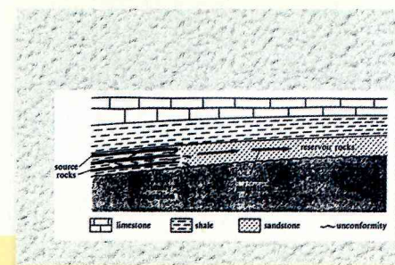
(fig D) De olie verzamelt zich in een ondergrondse holte (olieval) van waaruit die niet meer kan wegstromen. Gas is lichter dan olie en verzamelt zich erboven.
