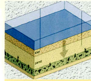
(fig A) Dode zeediertjes zinken naar de bodem.
